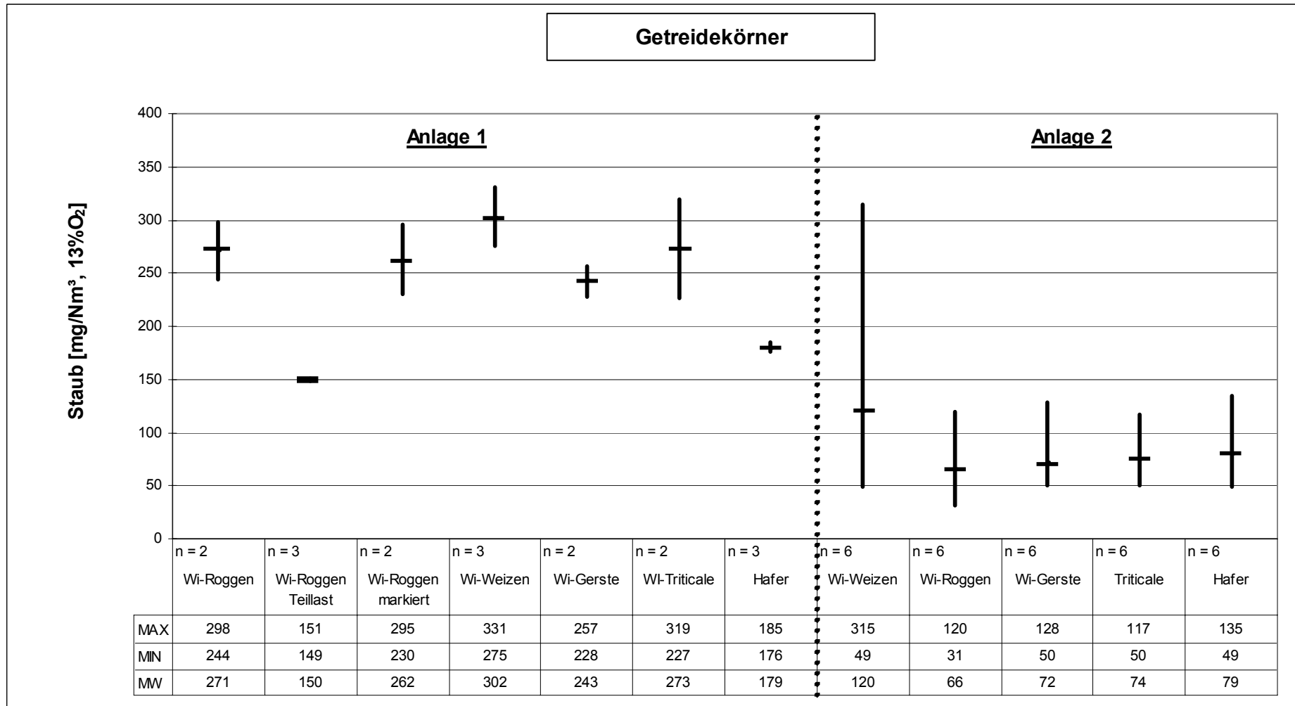
Abhängigkeit der Staubemissionen von der Verbrennungstechnik (unterschiedliche Anlagen) bei gleichem Brennstoff
